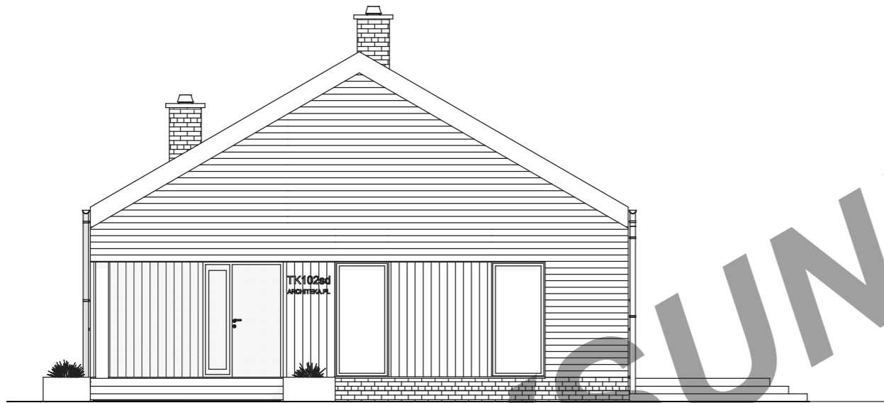
ELEWACJA FRONTOWA
