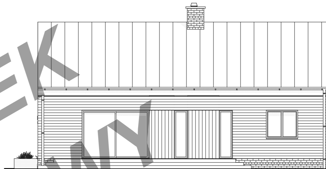
ELEWACJA OGRODOWA
